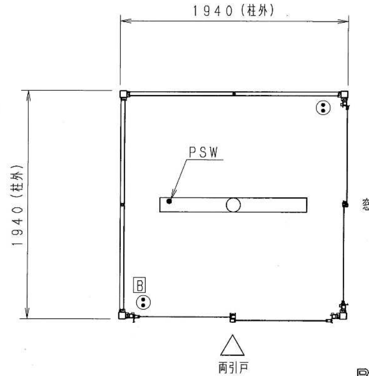
平面図
