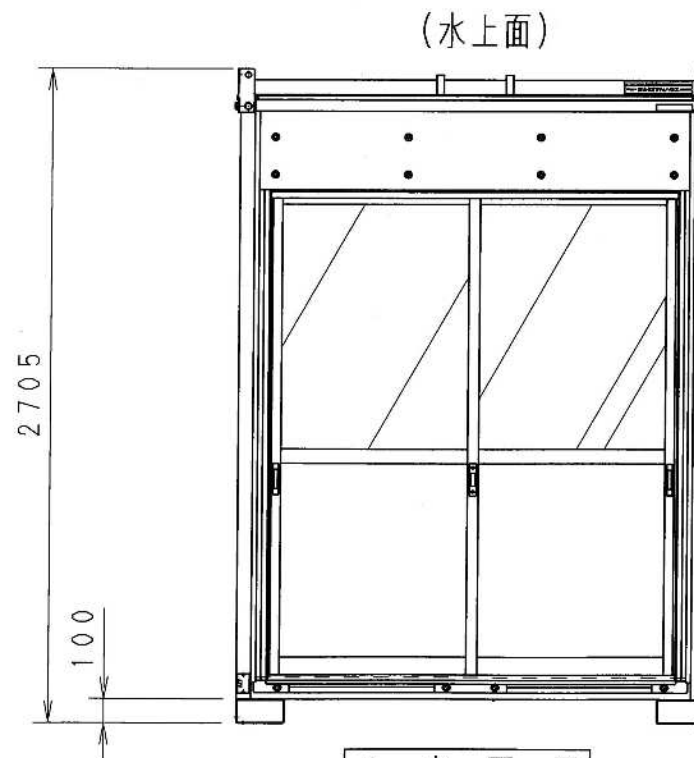
A 立面図
