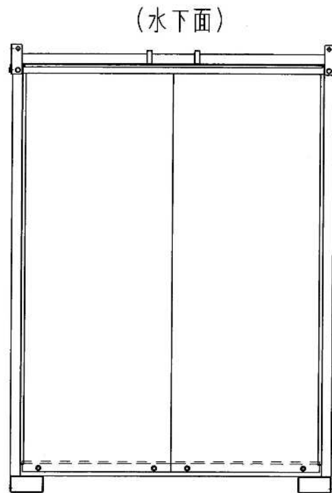
C 立面図
