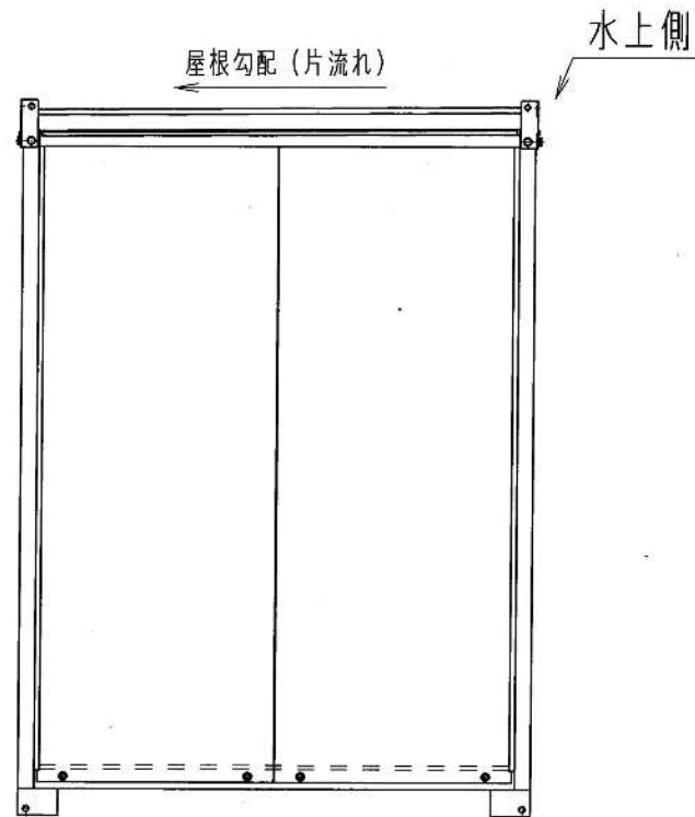
B 立面図
