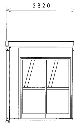
D 立面図 (妻面)
