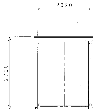
A 立面図 (桁面)
