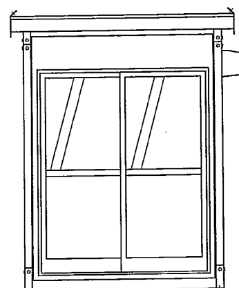
A 立面図
