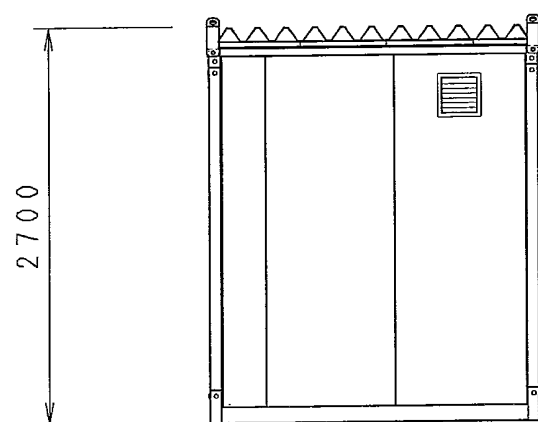
B 立面図
