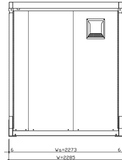
妻側 立面図
