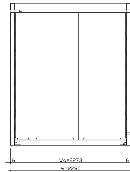
妻側 立面図
