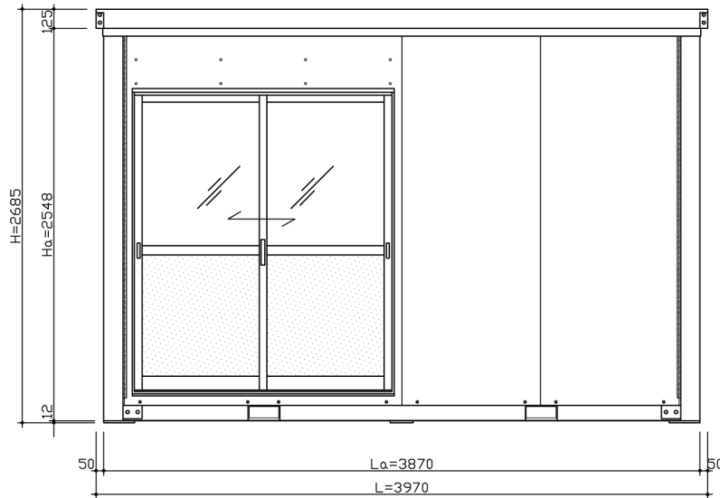
桁側 立面図
