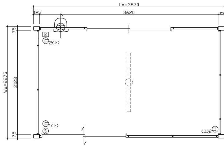
平面図
