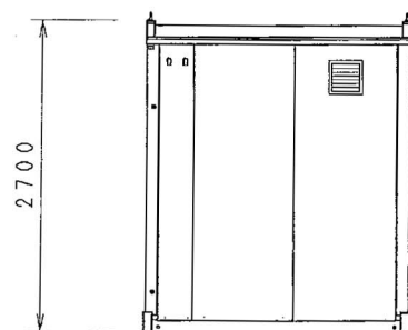
B 立面图
