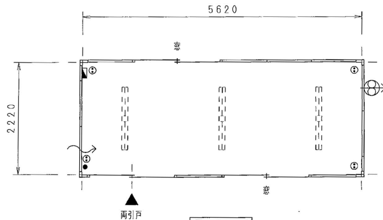
平面图
