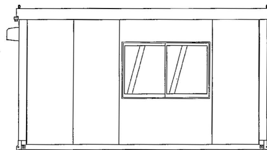
C 立面図
